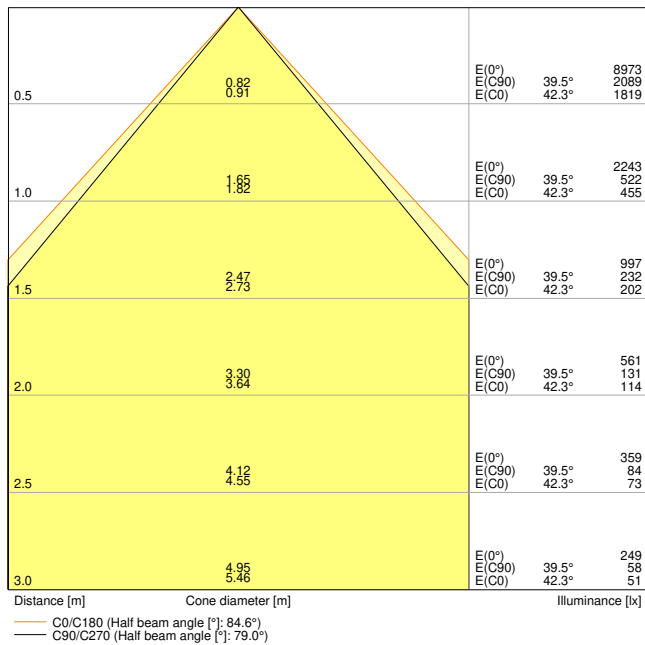
PL CMFT 600 P 33W 830 U19 DALIVR
